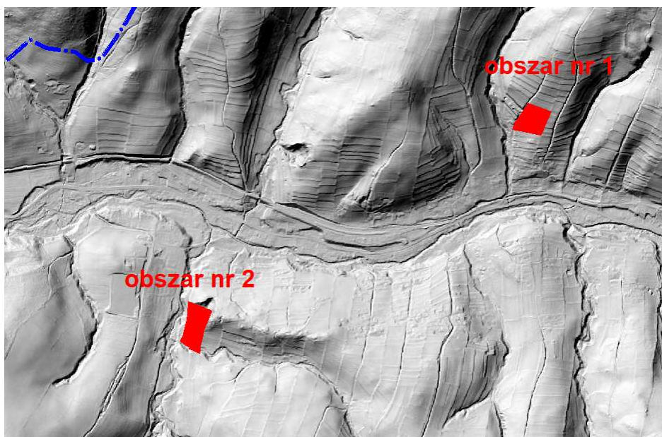
Ryc. 3. Rzeźba rejonu obszarów zmiany mpzp
