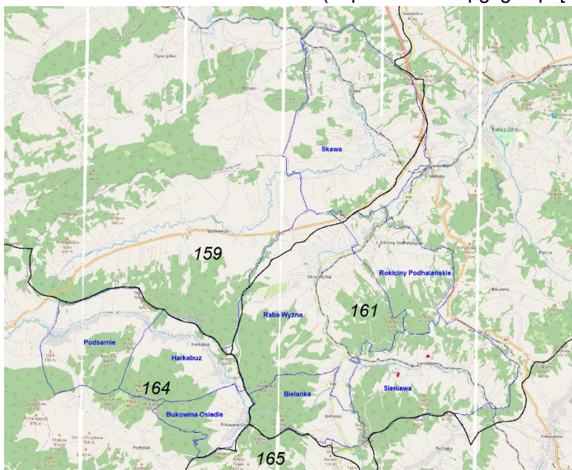
Ryc. 4. Położenie obszarów zmiany mpzp w obrębie JCWPd
